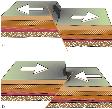
Dos tipos de fallas: a) normal, b) invertida.
