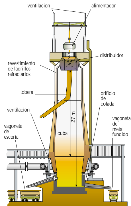
Esquema de los distintos componentes de un alto horno.
