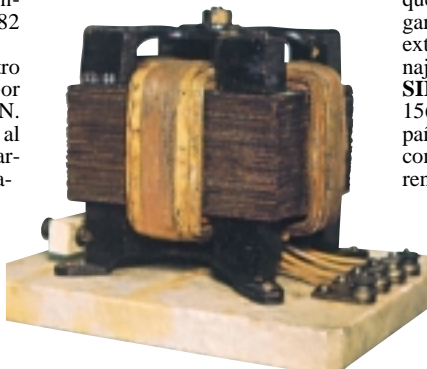
Transformador de silicio y acero (Museo de las Ciencias, Londres).
