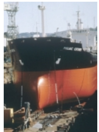
Reparar. Reparación de un barco en un dique seco.
