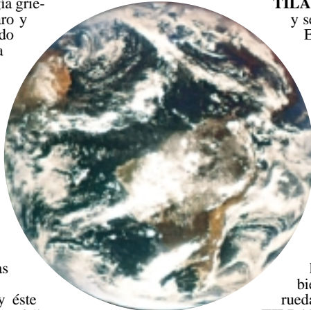
Imagen de la Tierra obtenida por el satélite ATS III.
