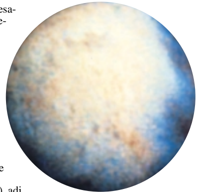
Imagen de Tritón , satélite de Neptuno.
