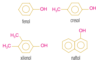
Fórmulas estructurales de algunos fenoles .
