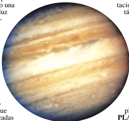
Júpiter es un planeta del Sistema Solar.
