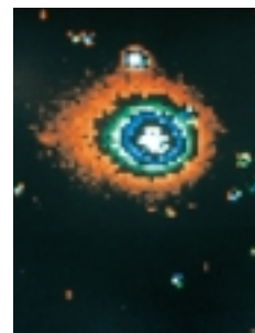
Los cometas son cuerpos celestes.
