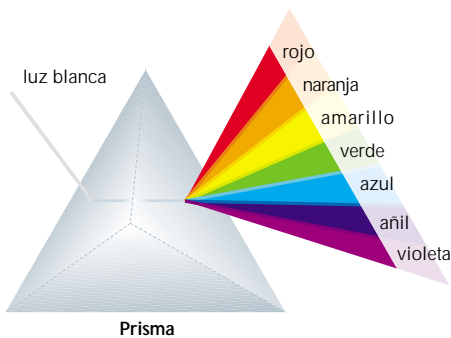
Descomposición de la luz blanca al atravesar un prisma óptico.
