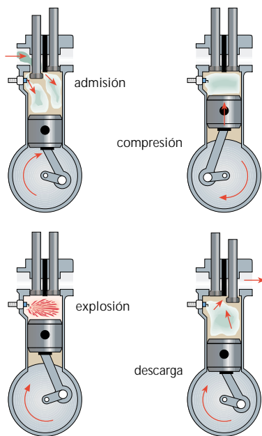
Esquema de las distintas fases del motor de explosión de cuatro tiempos.
