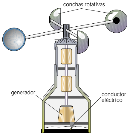
Esquema estructural de un anemómetro.
