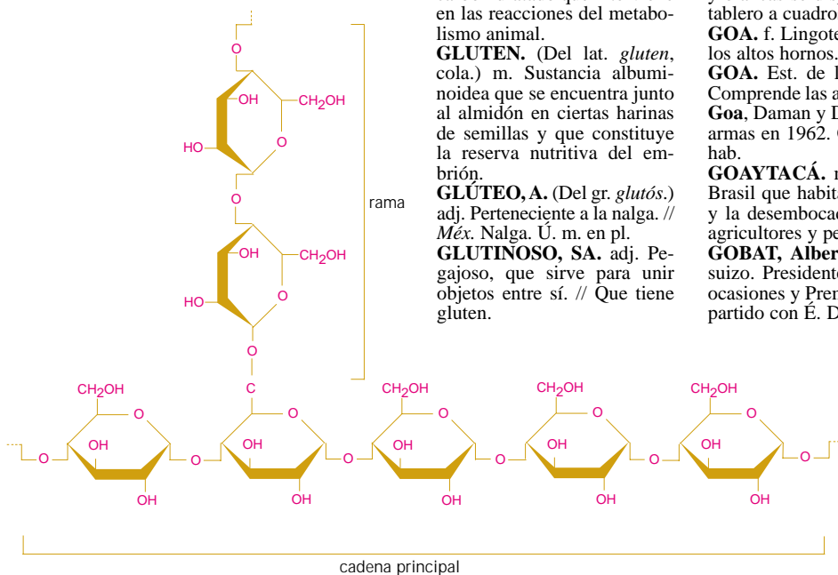
Fórmula estructural del glucógeno .
