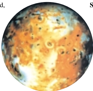
Fotografía de lo, satélite de Júpiter, tomada desde el Voyager 1 .
