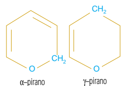
Fórmulas estructurales de dos isómeros del pirano.
