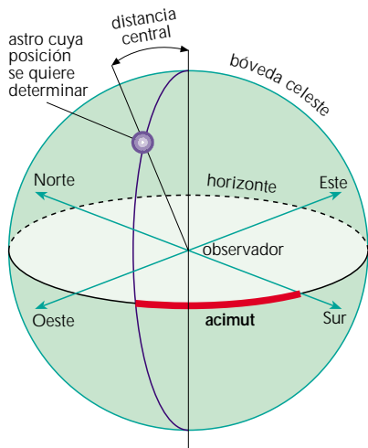
Esquema de coordenadas celestes, a partir de las cuales se determina el acimut de un astro.
