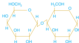
Fórmula estructural de la lactosa .
