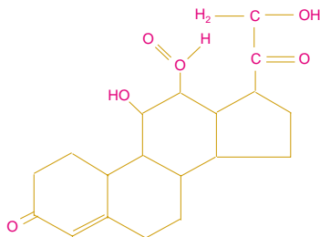
Fórmula estructural de la aldosterona .
