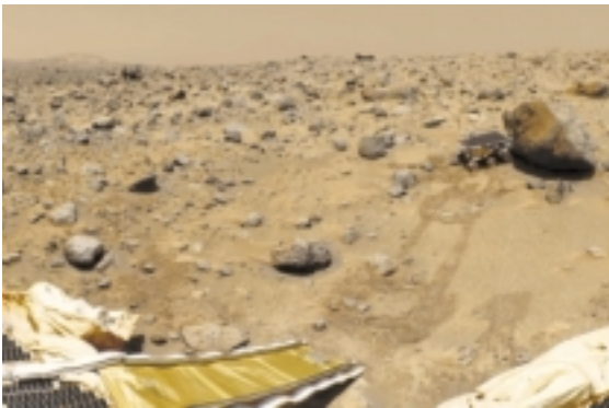
Imagen del planeta Marte enviada por la sonda Mars Pathfinder en 1997.
