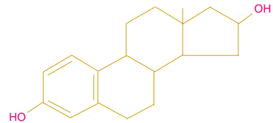
Fórmula estructural del estrógeno.
