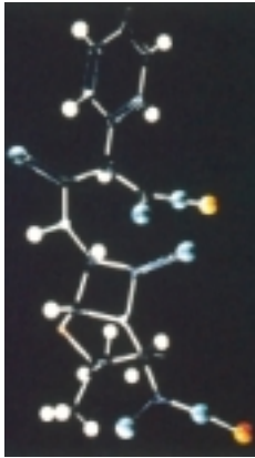
Modelo de estructura de una molécula.
