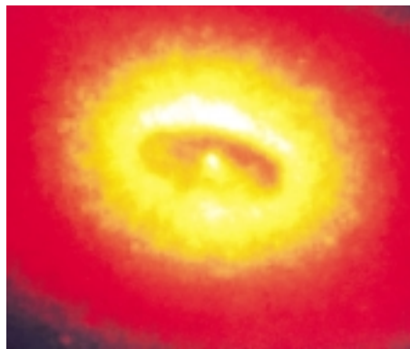
Imagen de un agujero negro obtenida por el telescopio espacial Hubble.
