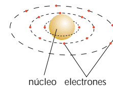
MODELO ATÓMICO DE BOHR
