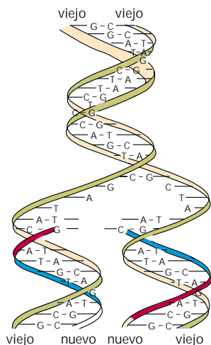
Ilustración del desdoblamiento de las bases que integran la espiral del ADN (A, T, C y G) para constituir dos nuevas cadenas helicoidales.
