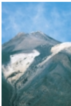
Ceniza volcánica perteneciente al Teide, en Tenerife, España.
