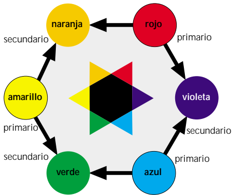
Esquema representativo de los colores primarios y secundarios.
