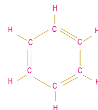
Fórmula estructural del benceno .
