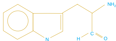
Fórmula estructural del triptófano.
