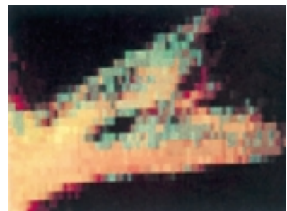
Imagen espectroscópica de una protuberancia solar.
